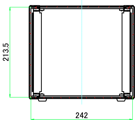
B-B ( 1 : 5.5 )
