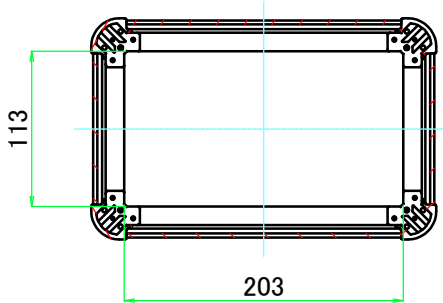
C-C ( 1 : 5.5 )
