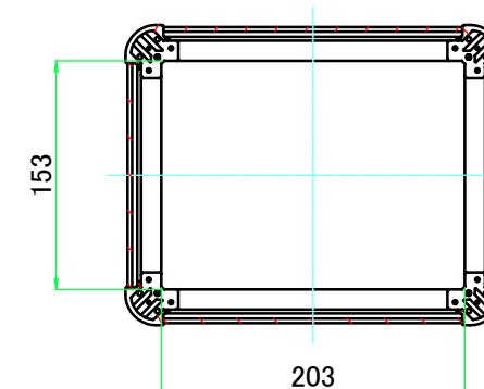
C-C ( 1 : 5.5 )
