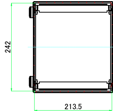
A-A (1:6)
