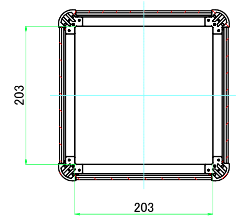
C-C ( 1 : 5.5 )
