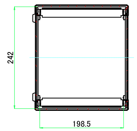
A-A ( 1 : 5.5 )
