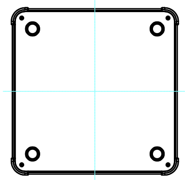
C-C ( 1 : 5.5 )
