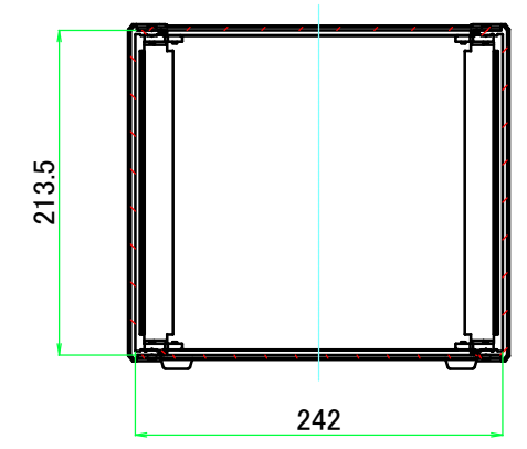
B-B ( 1 : 5.5 )
