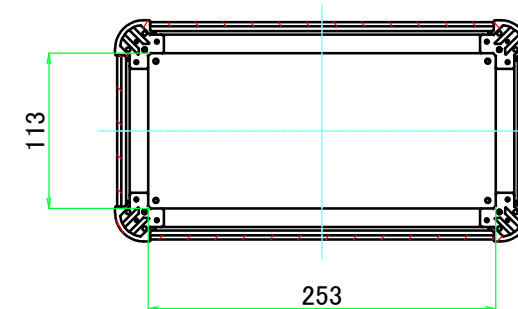
C-C ( 1 : 5.5 )
