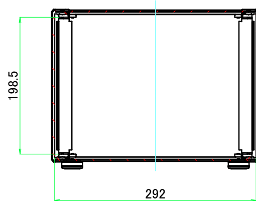
B-B ( 1 : 5.5 )
