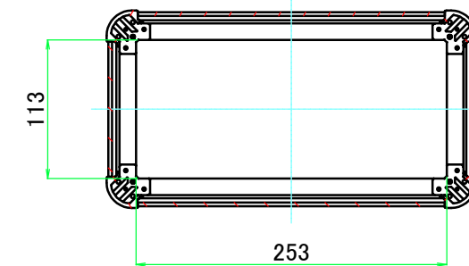
C-C ( 1 : 5.5 )
