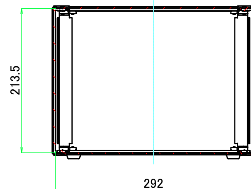
B-B ( 1 : 5.5 )
