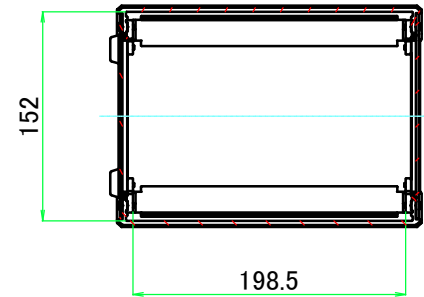
A-A ( 1 : 5.5 )
