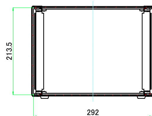
B-B ( 1 : 5.5 )
