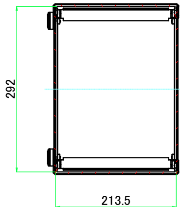
A-A ( 1 : 6.5 )
