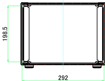
B-B ( 1 : 6.5 )
