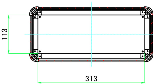
C-C ( 1 : 6.5 )
