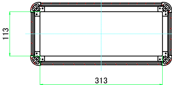
C-C ( 1 : 6 )
