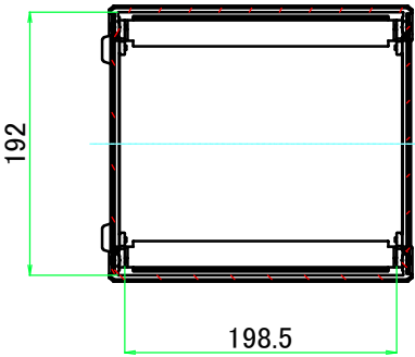
A-A ( 1 : 6 )
