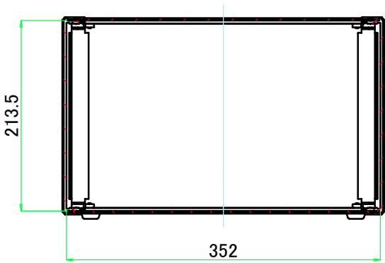
B-B ( 1 : 6 )
