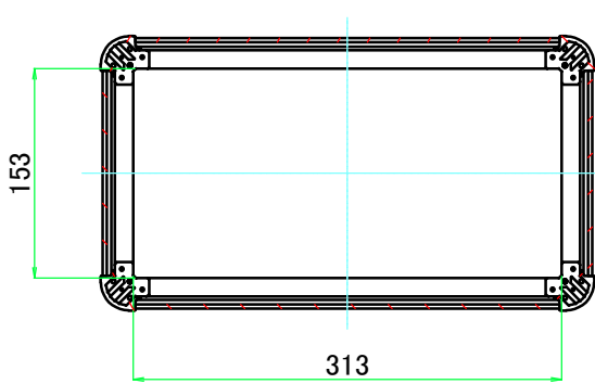
C-C ( 1 : 6 )
