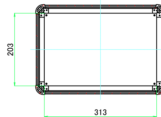
C-C ( 1 : 6.5 )
