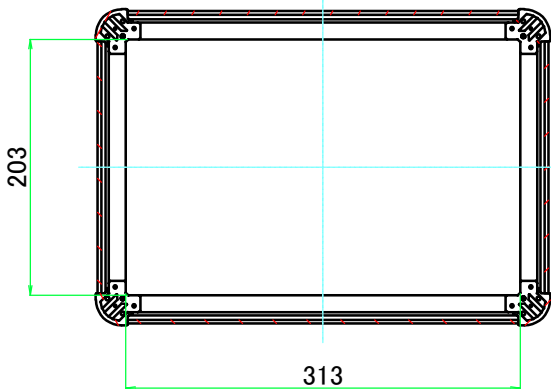
C-C ( 1 : 6 )
