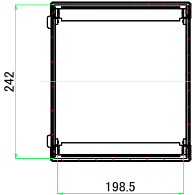
A-A ( 1 : 6 )
