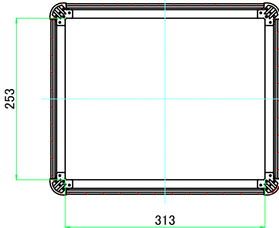
C-C ( 1 : 6 )
