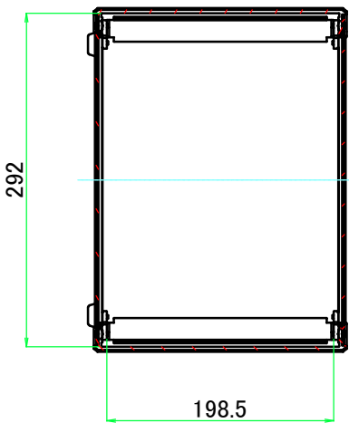
A-A ( 1 : 6 )
