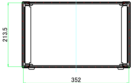
B-B ( 1 : 6 )
