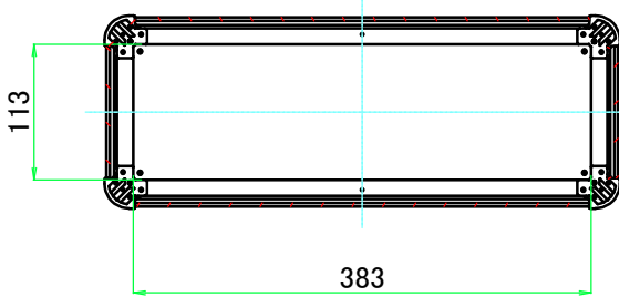
C-C ( 1 : 7 )
