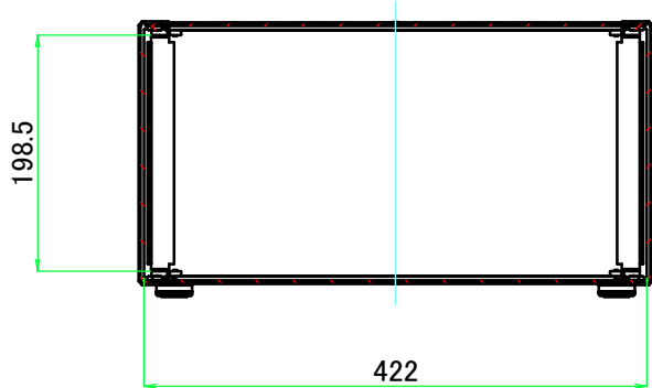
B-B ( 1 : 7 )
