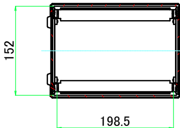
A-A ( 1 : 6.5 )
