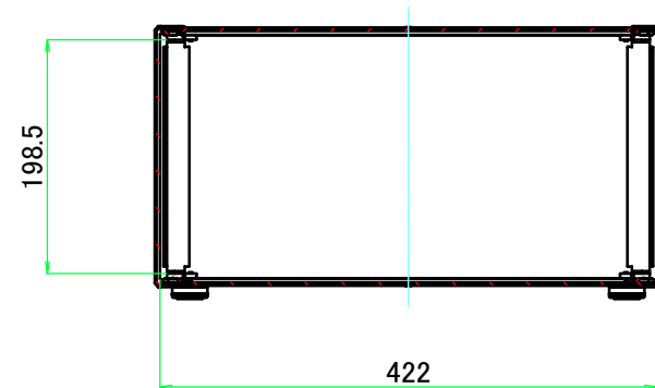
B-B ( 1 : 7 )
