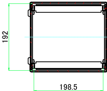
A-A ( 1 : 6.5 )
