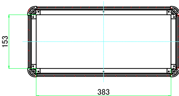
C-C ( 1 : 6.5 )
