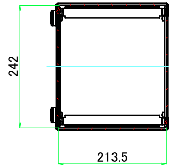
A-A ( 1 : 7.5 )
