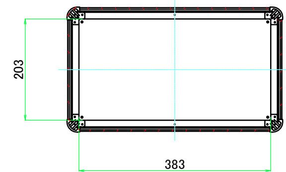
C-C ( 1 : 7.5 )
