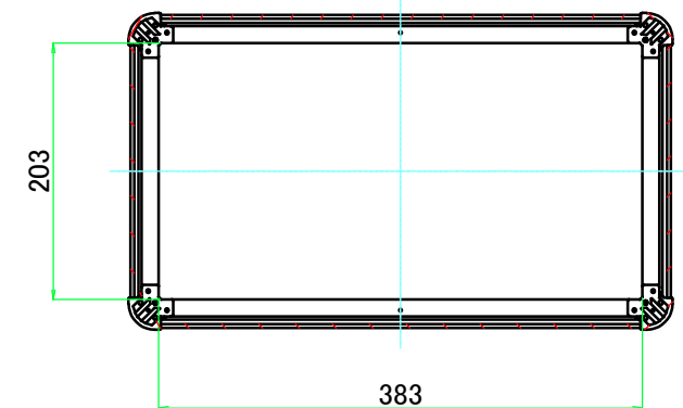
C-C ( 1 : 6.5 )
