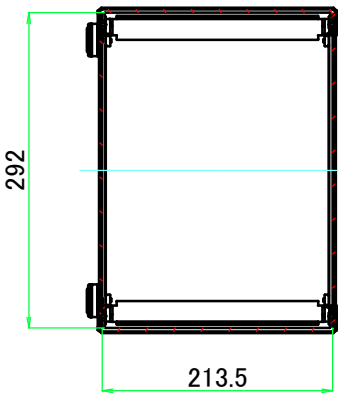
A-A (1:7)
