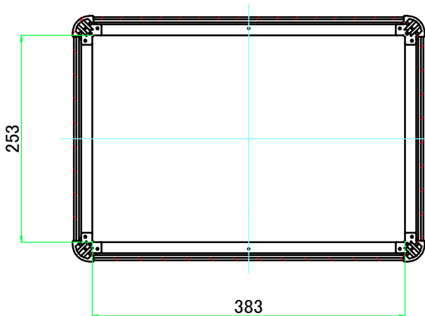
C-C ( 1 : 6.5 )
