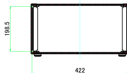
B-B ( 1 : 8 )
