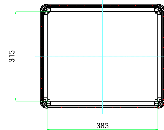
C-C ( 1 : 8 )
