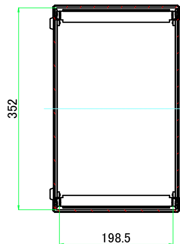
A-A ( 1 : 6.5 )
