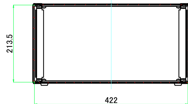
B-B ( 1 : 6.5 )
