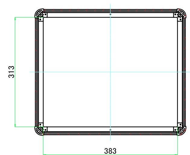
C-C ( 1 : 6.5 )
