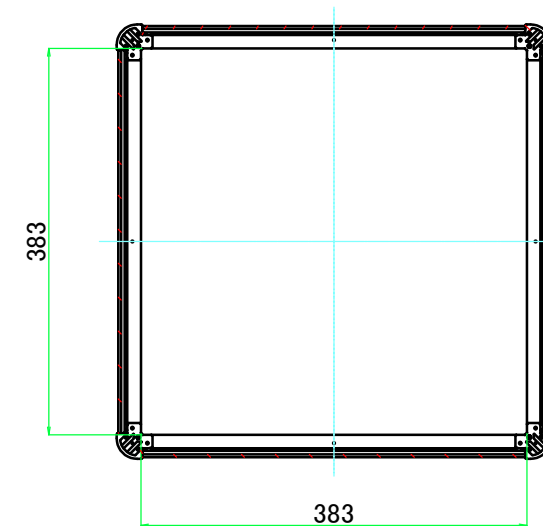
C-C ( 1 : 7.5 )
