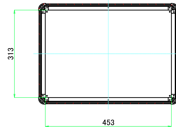
C-C ( 1 : 8 )
