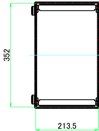
A-A ( 1 : 8 )
