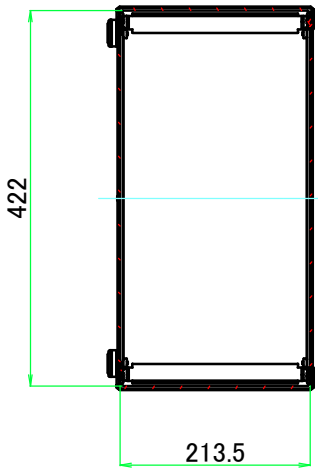
A-A ( 1 : 8.5 )
