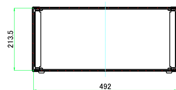
B-B ( 1 : 7.5 )
