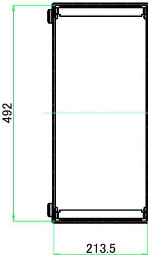
A-A ( 1 : 8.5 )
