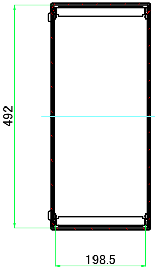
A-A ( 1 : 8.5 )
