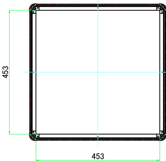
C-C ( 1 : 8.5 )
