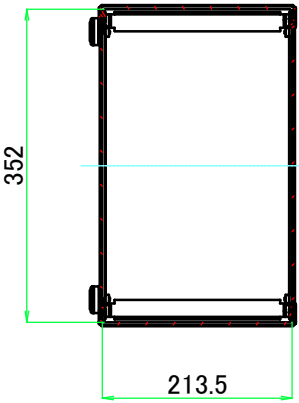
A-A ( 1 : 8.5 )
