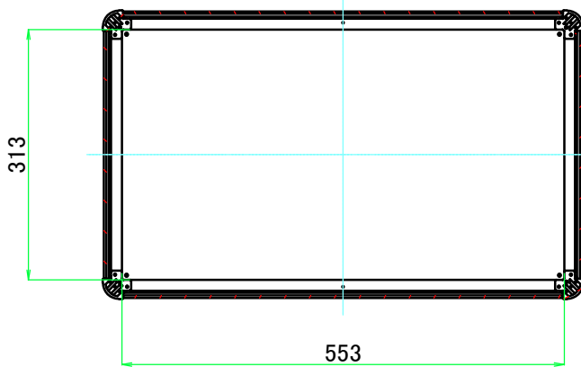
C-C ( 1 : 8.5 )
