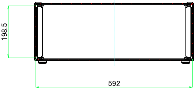
B-B ( 1 : 8.5 )
