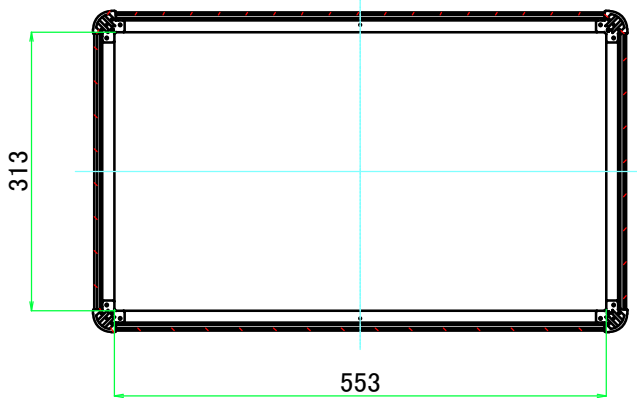
C-C ( 1 : 8.5 )
