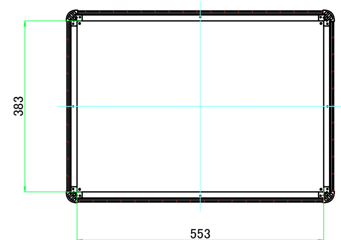
C-C ( 1 : 8.5 )
