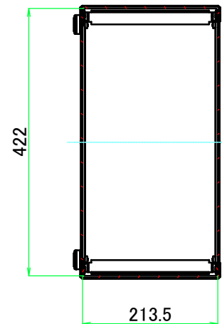
A-A ( 1 : 8.5 )
