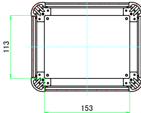
C-C ( 1 : 4 )
