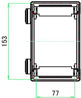
A-A ( 1 : 4 )
