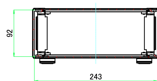
B-B ( 1 : 4.5 )
