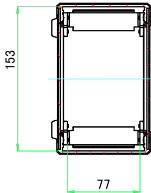
A-A (1:4)
