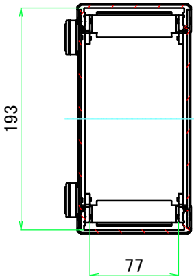
A-A ( 1 : 4.5 )
