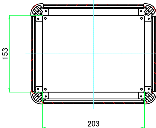
C-C ( 1 : 4.5 )
