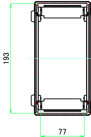
A-A (1:4)
