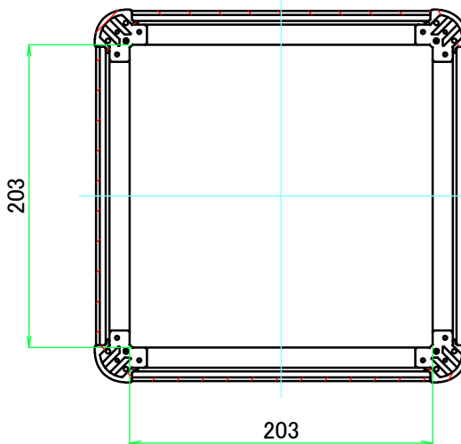
C-C ( 1 : 4.5 )
