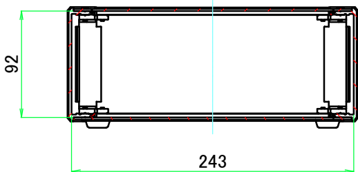
B-B ( 1 : 4.5 )
