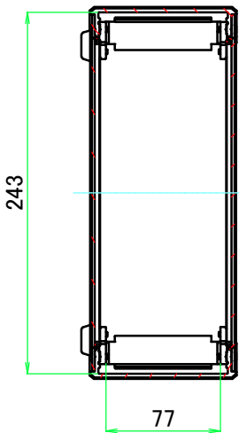
A-A ( 1 : 4.5 )
