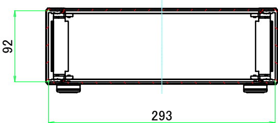
B-B ( 1 : 5 )
