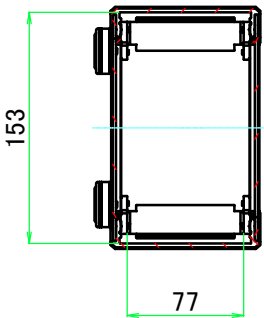
A-A ( 1 : 5 )
