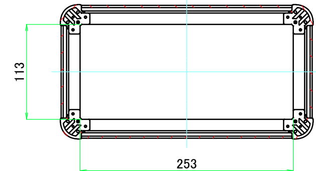
C-C ( 1 : 4.5 )
