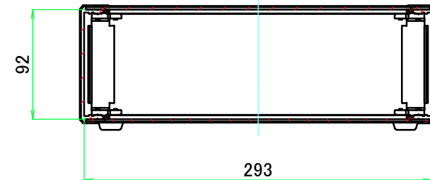
B-B ( 1 : 4.5 )
