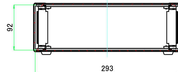
B-B ( 1 : 4.5 )
