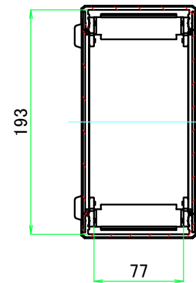
A-A ( 1 : 4.5 )
