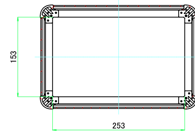
C-C ( 1 : 4.5 )
