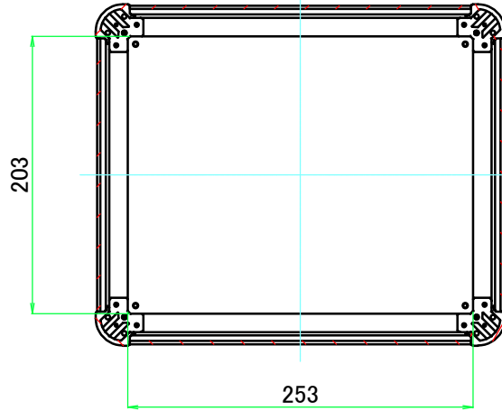
C-C ( 1 : 5 )
