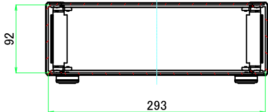
B-B ( 1 : 5 )
