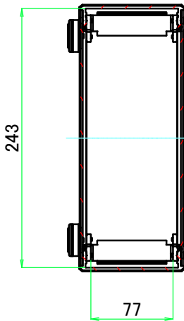
A-A ( 1 : 5 )
