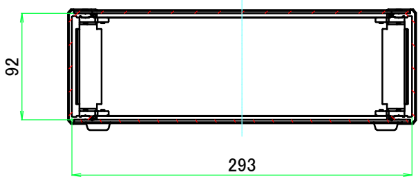
B-B ( 1 : 4.5 )
