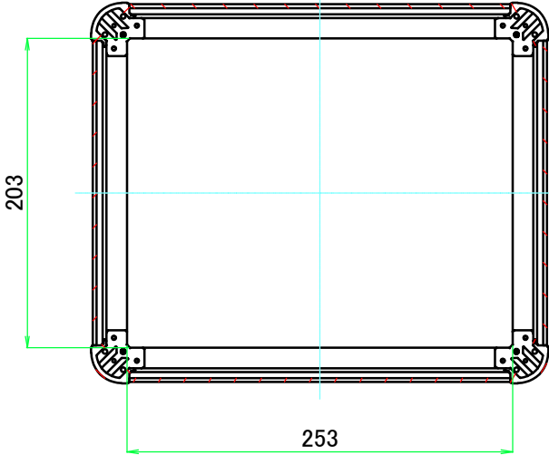
C-C ( 1 : 4.5 )
