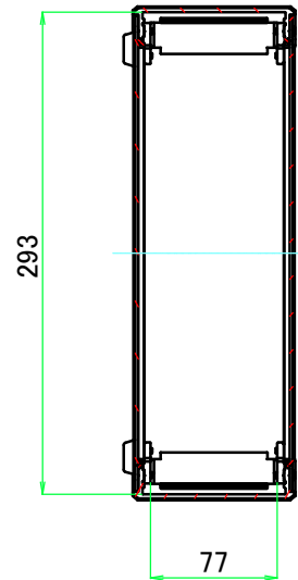
A-A ( 1 : 5 )
