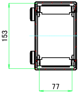
A-A ( 1 : 5 )
