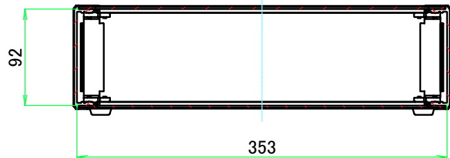
B-B ( 1 : 5 )
