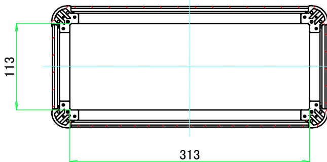
C-C ( 1 : 5 )
