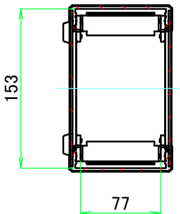
A-A ( 1 : 5 )
