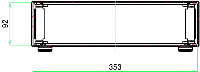
B-B ( 1 : 5 )
