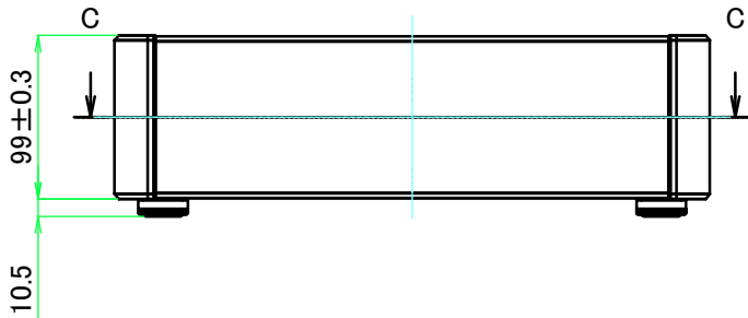
B-B ( 1 : 5 )
