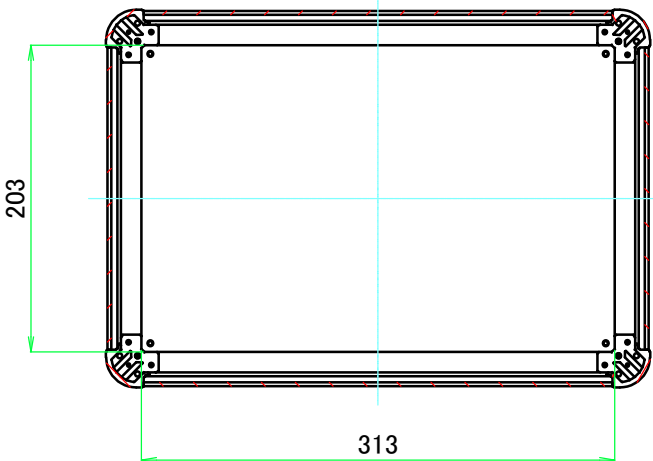
C-C ( 1 : 5 )
