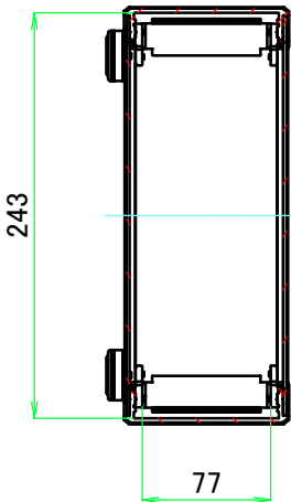
A-A ( 1 : 5 )
