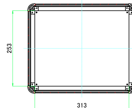
C-C ( 1 : 6 )
